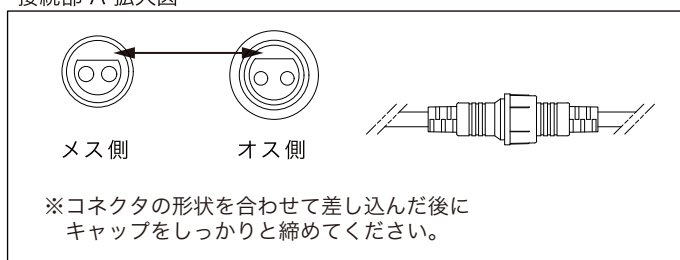
接続部 A 拡大図
